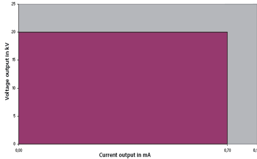
Stromversorgung Ausgang
